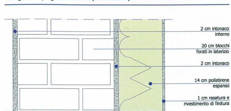
stratigrafia di progetto del muro perimetrale tipo
