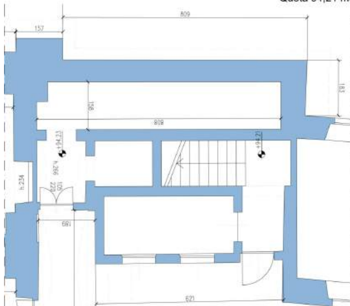
CORPO 9 PIANTA PIANO TERRA Quota 94,21 mt
