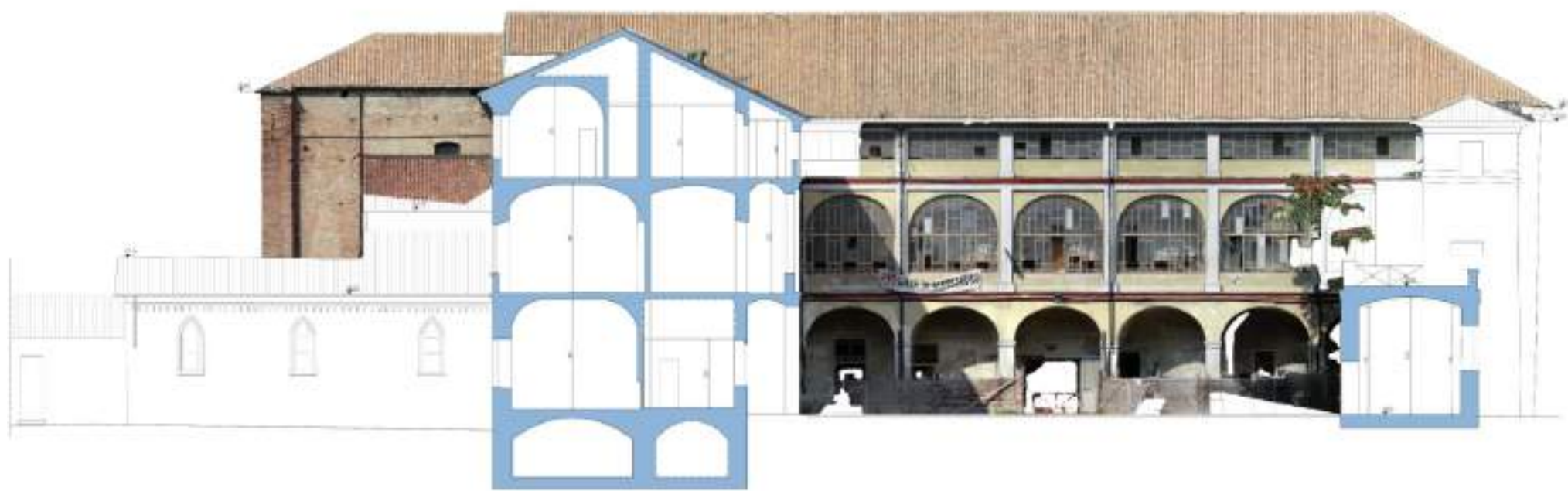
PROSPETTO SUD EST CORPO I - CORPO II
