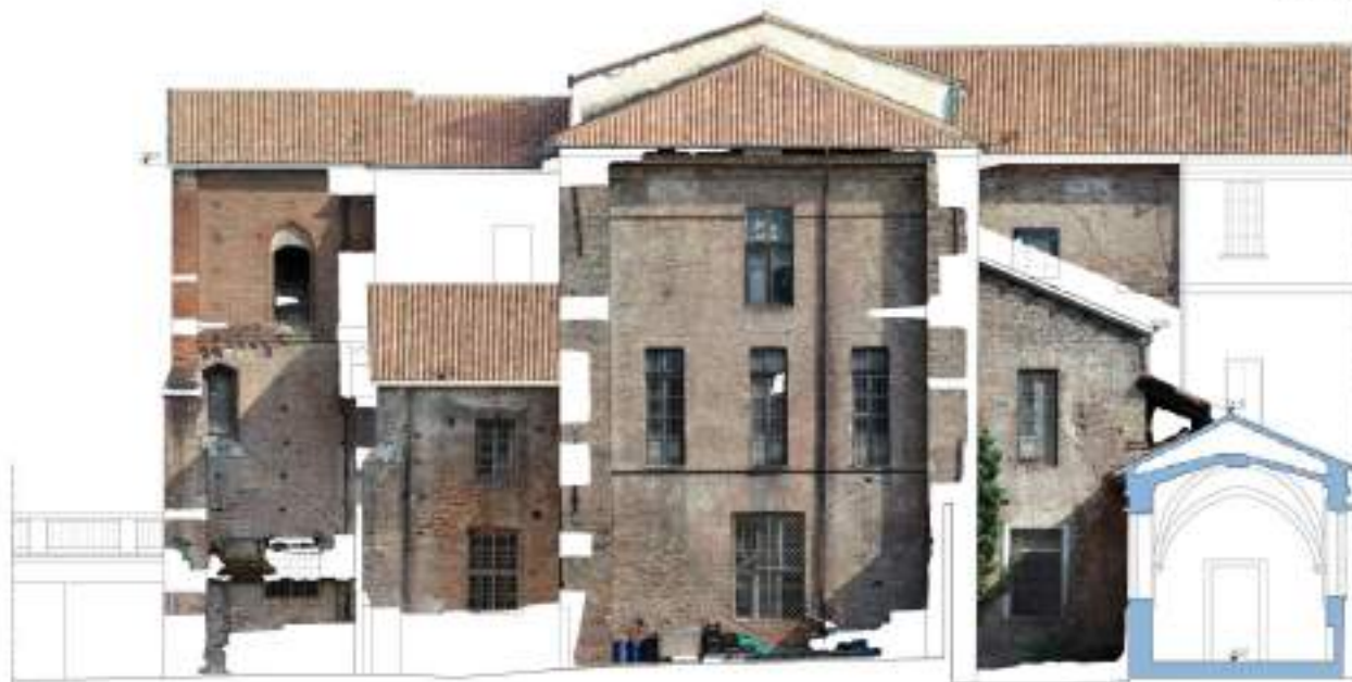
PROSPETTO SUD OVEST CORPO 1
