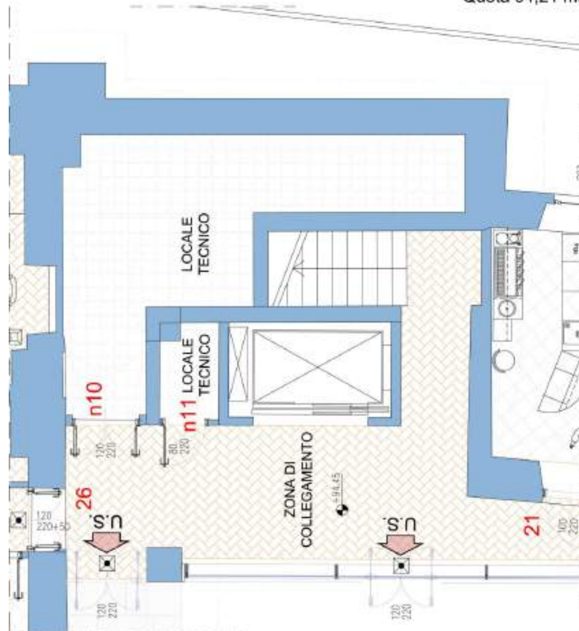
CORPO 9 PIANTA PIANO TERRA Quota 94,21 mt
