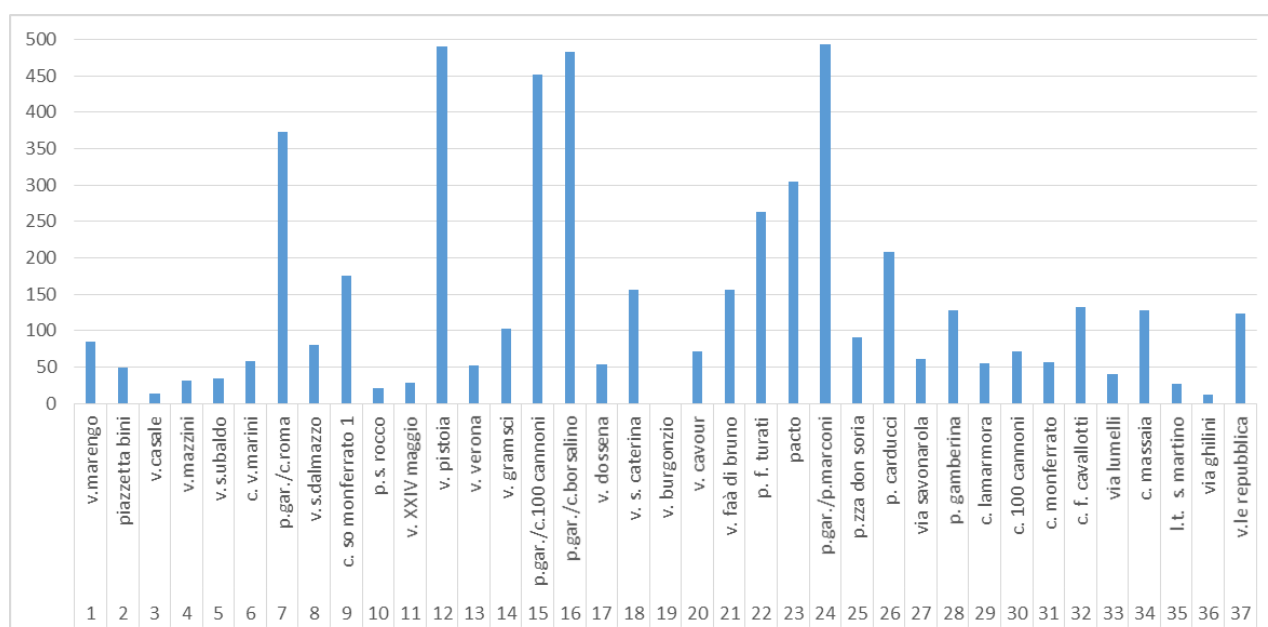
Figura 5-5: Ore giornaliere di utilizzo spazi di sosta tariffati per parcometro (media giornaliera, aprile 2016)
