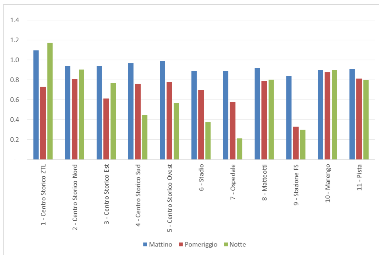
Figura 5-4: Domanda di sosta: coefficiente di occupazione (mattino, pomeriggio, notte)
