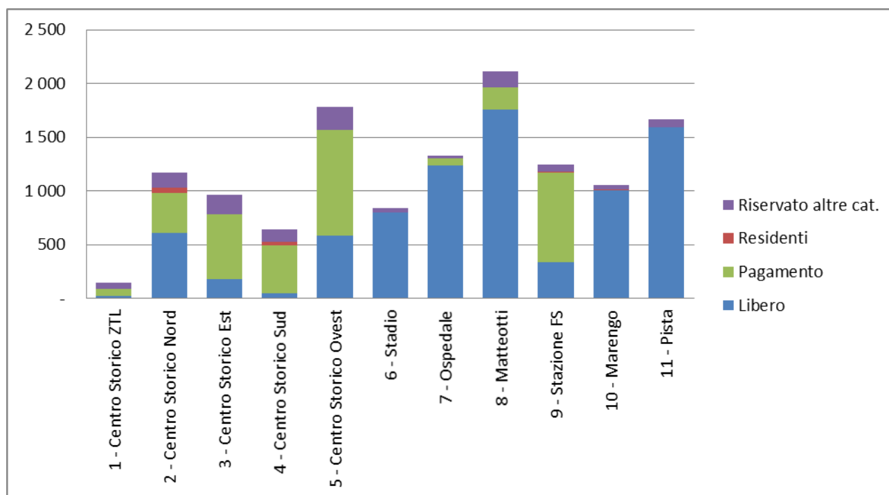
Figura 5-2: Offerta di sosta per ambito e tipologia
