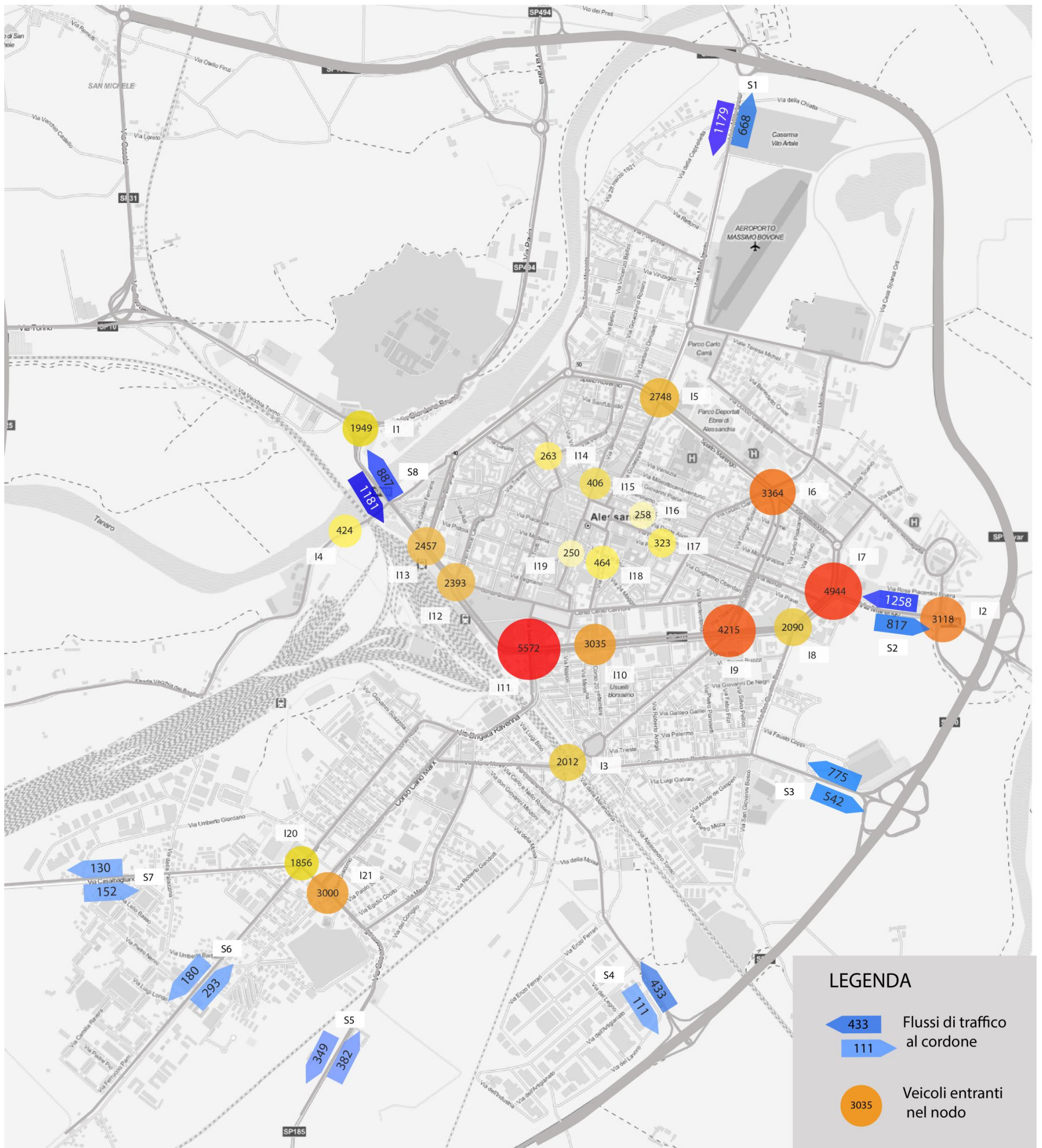
Figura 4-6: Flussi di traffico nell'ora di punta della mattina
