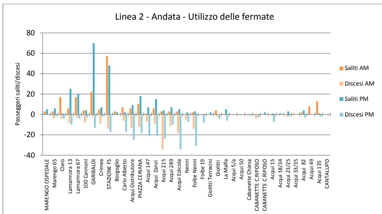
Figura 4-21: Media passeggeri a bordo. Corse di andata. Linea 2
