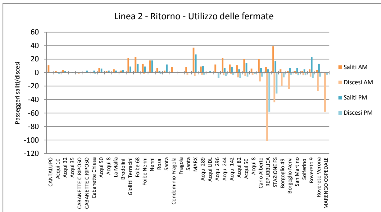
Figura 4-23: Media passeggeri a bordo. Corse di ritorno. Linea 2
