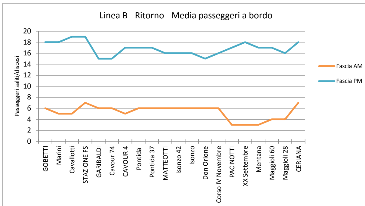
Figura 4-18: Media passeggeri a bordo. Corse di ritorno. Linea B
