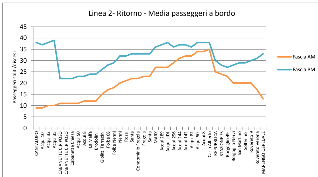
Figura 4-22: Utilizzo fermate. Totale passeggeri corse di ritorno per fascia oraria. Linea 2
