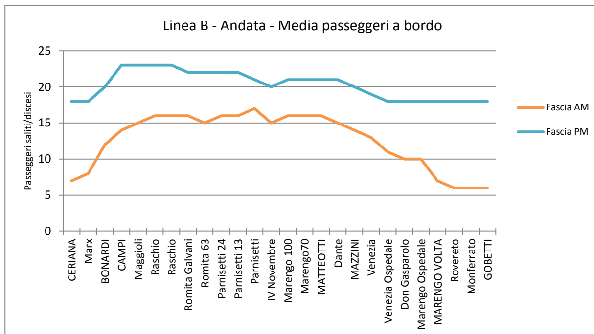
Figura 4-16: Media passeggeri a bordo. Corse di andata. Linea B
