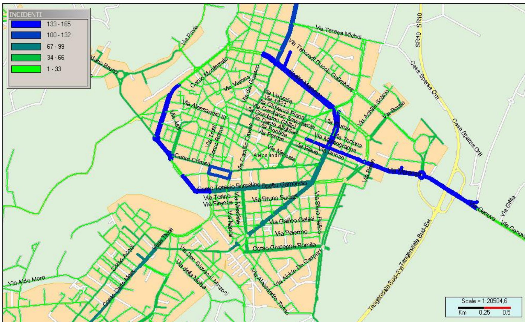
Figura 6-1: Sinistrosità per via, periodo 01/01/2013 - 31/05/2016: area centro cittadino
