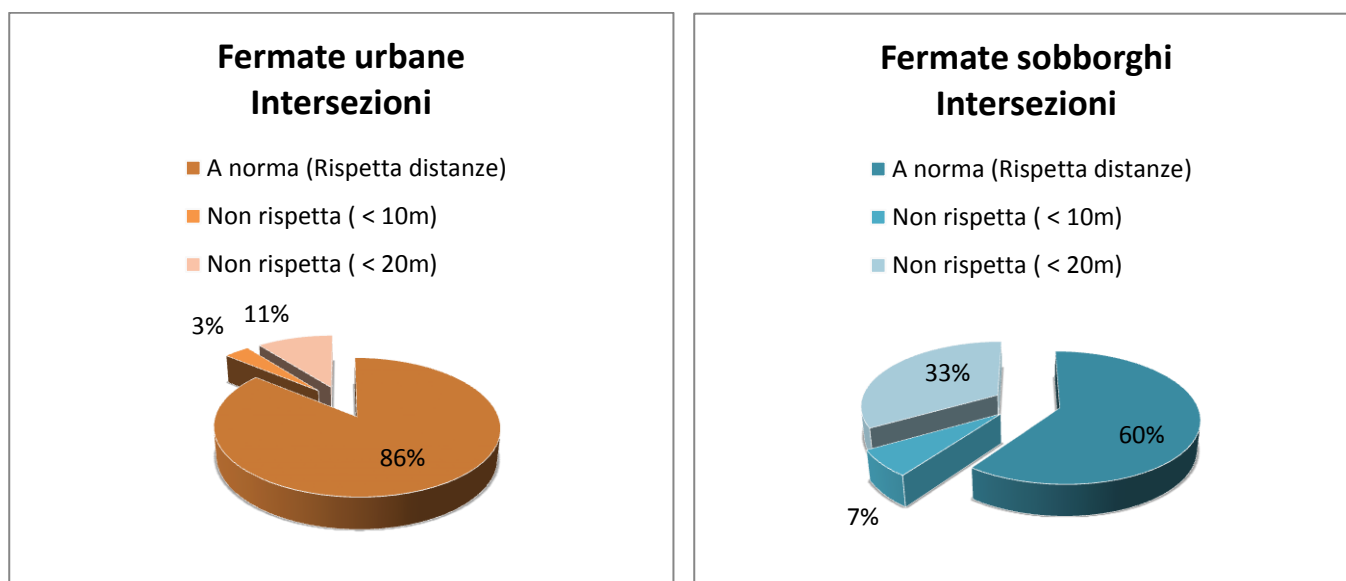
Figura 3-9: Allestimento delle fermate: posizione della fermata rispetto all'intersezione
