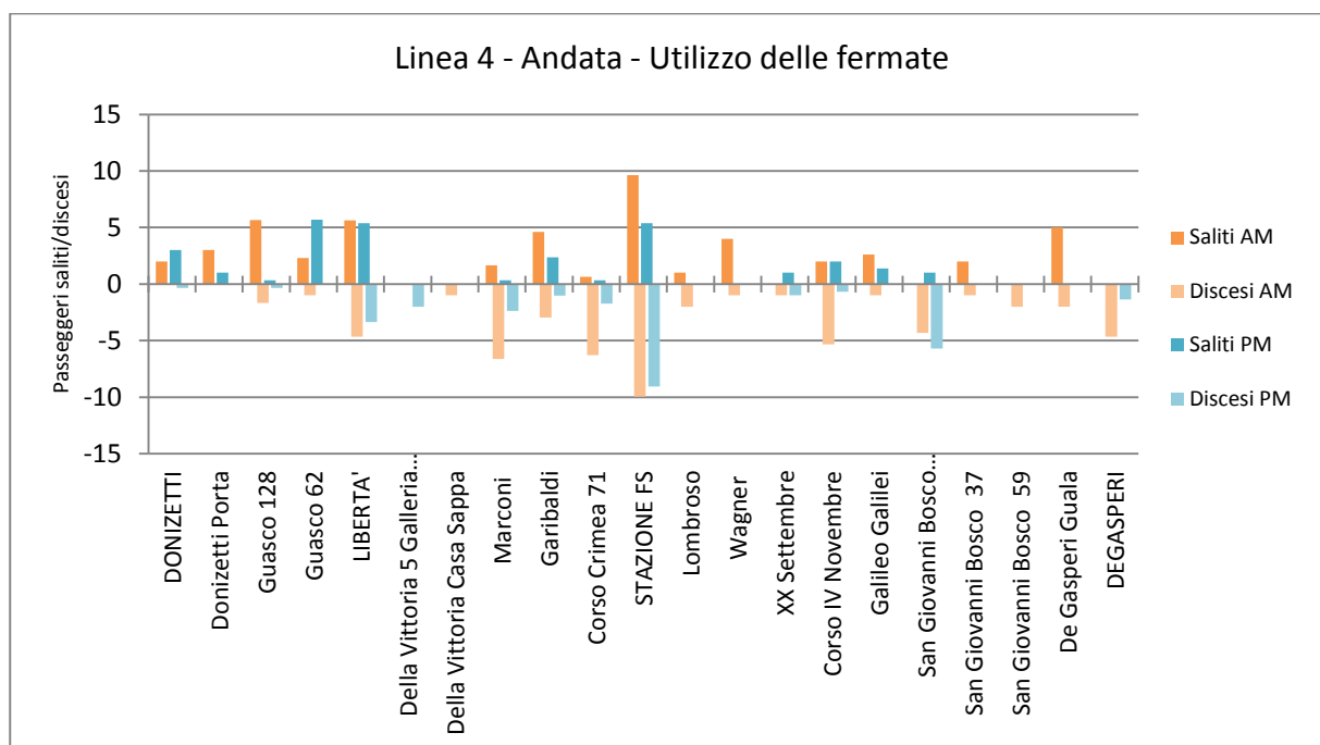
Figura 4-29: Media passeggeri a bordo. Corse di andata. Linea 4
