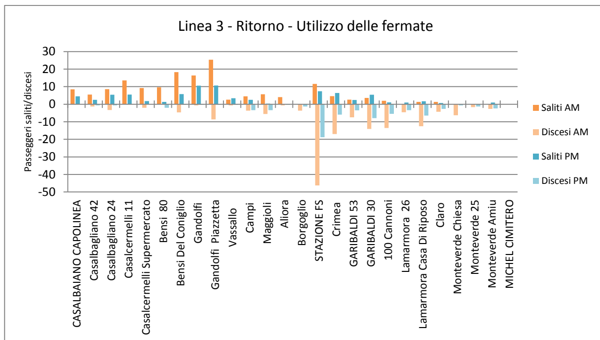
Figura 4-27: Media passeggeri a bordo. Corse di ritorno. Linea 3
