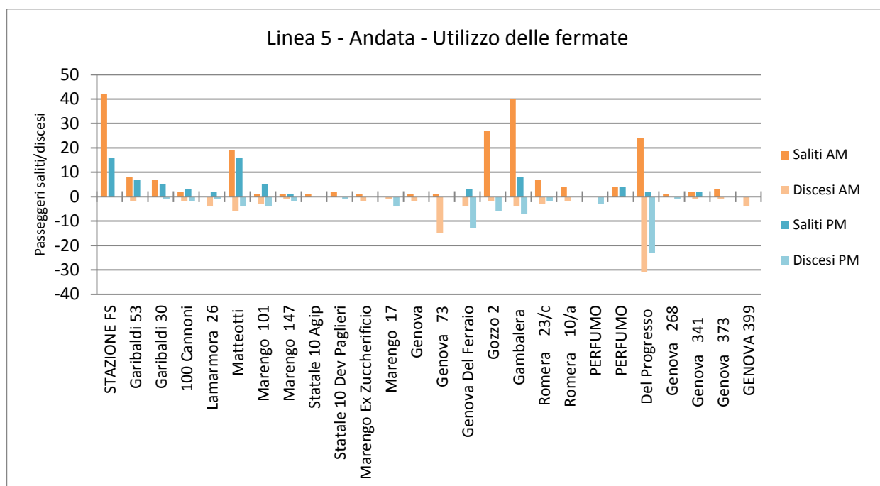
Figura 4-33: Media passeggeri a bordo. Corse di andata. Linea 5
