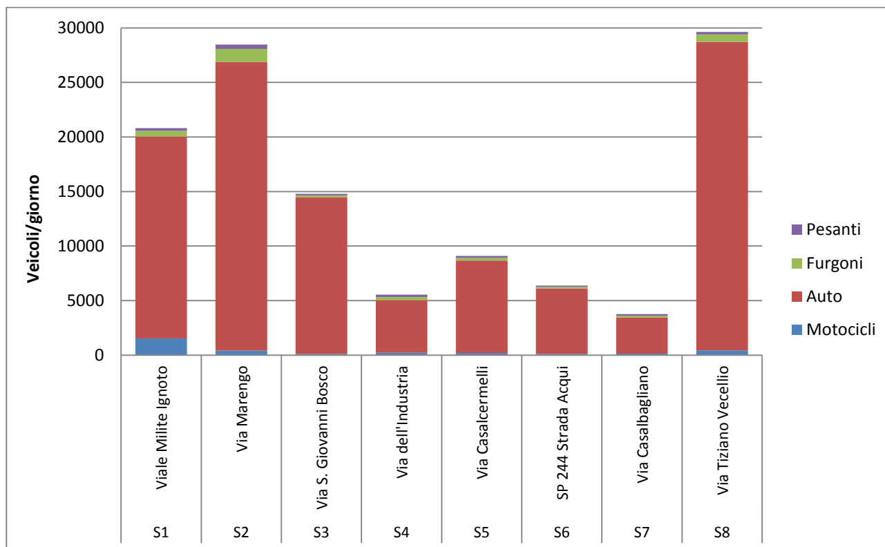
Figura 4-7: Flussi di traffico totali al cordone (veicoli/giorno). Traffico giornaliero medio
