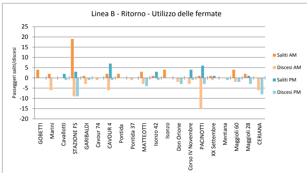
Figura 4-19: Utilizzo fermate. Totale passeggeri corse di ritorno per fascia oraria. Linea B
