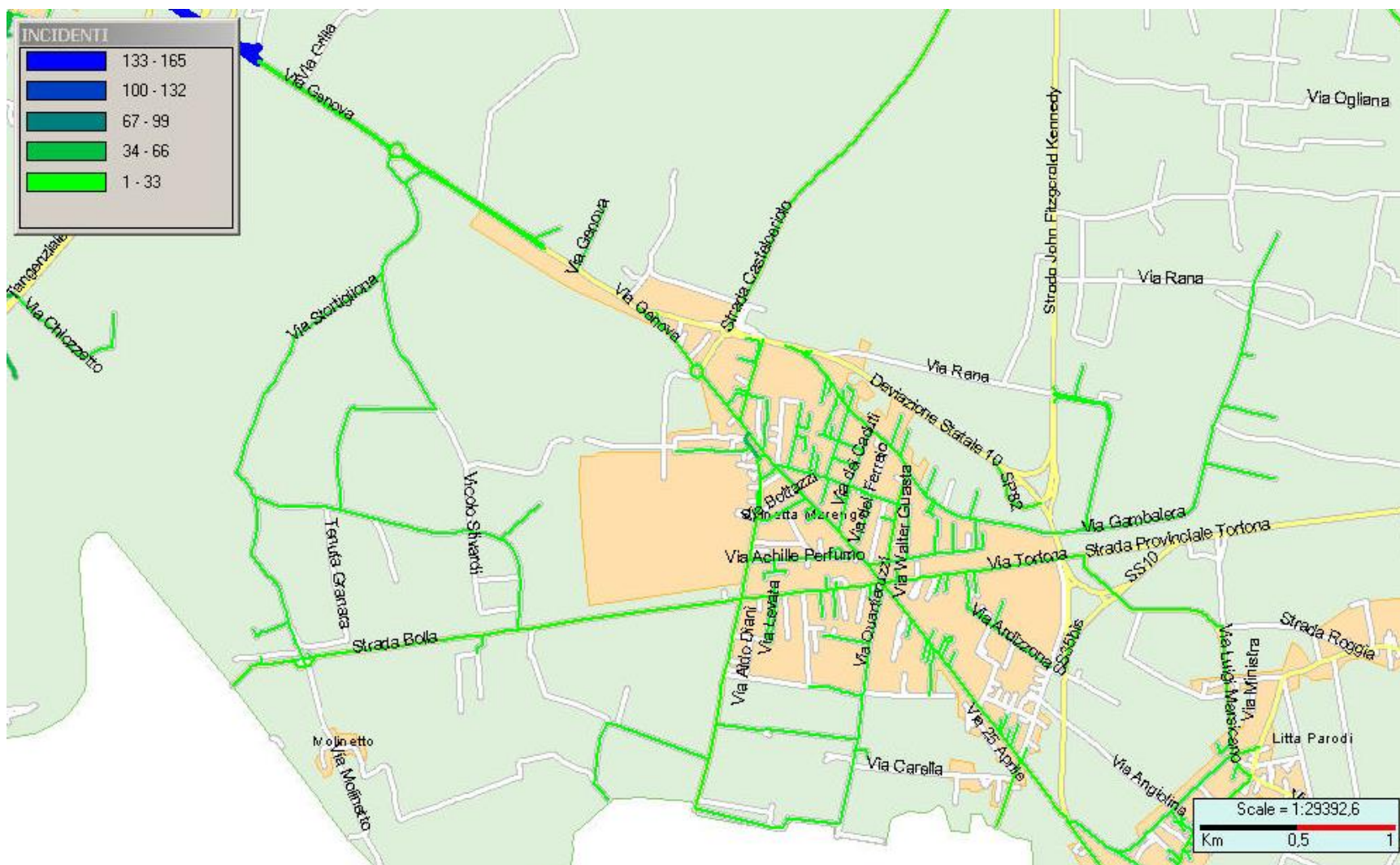
Figura 6-8: Sinistrosità per via, periodo 01/01/2013 - 31/05/2016: Spinetta Marengo
