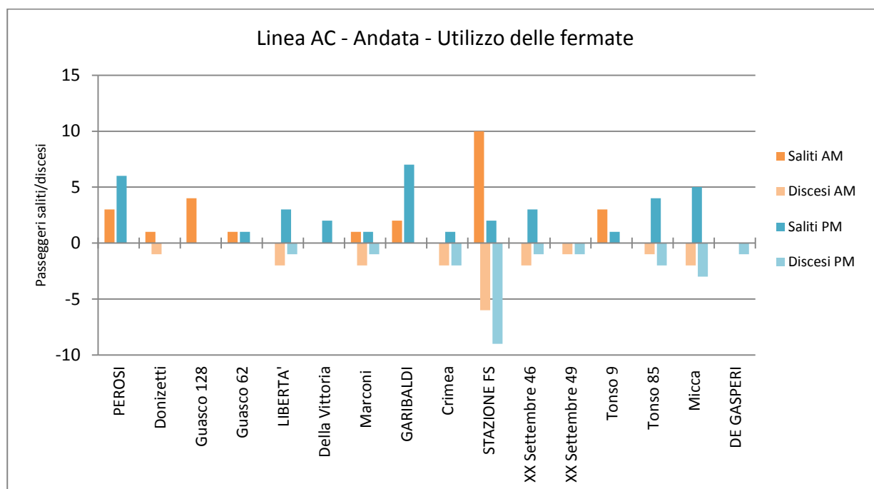
Figura 4-13: Utilizzo fermate. Totale passeggeri corse di andata per fascia oraria. Linea A/C
