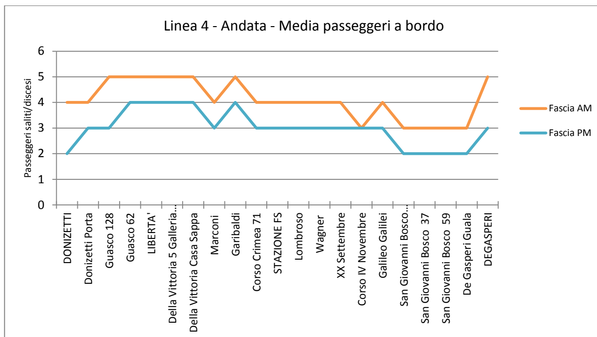
Figura 4-28: Utilizzo fermate. Totale passeggeri corse di andata per fascia oraria. Linea 4
