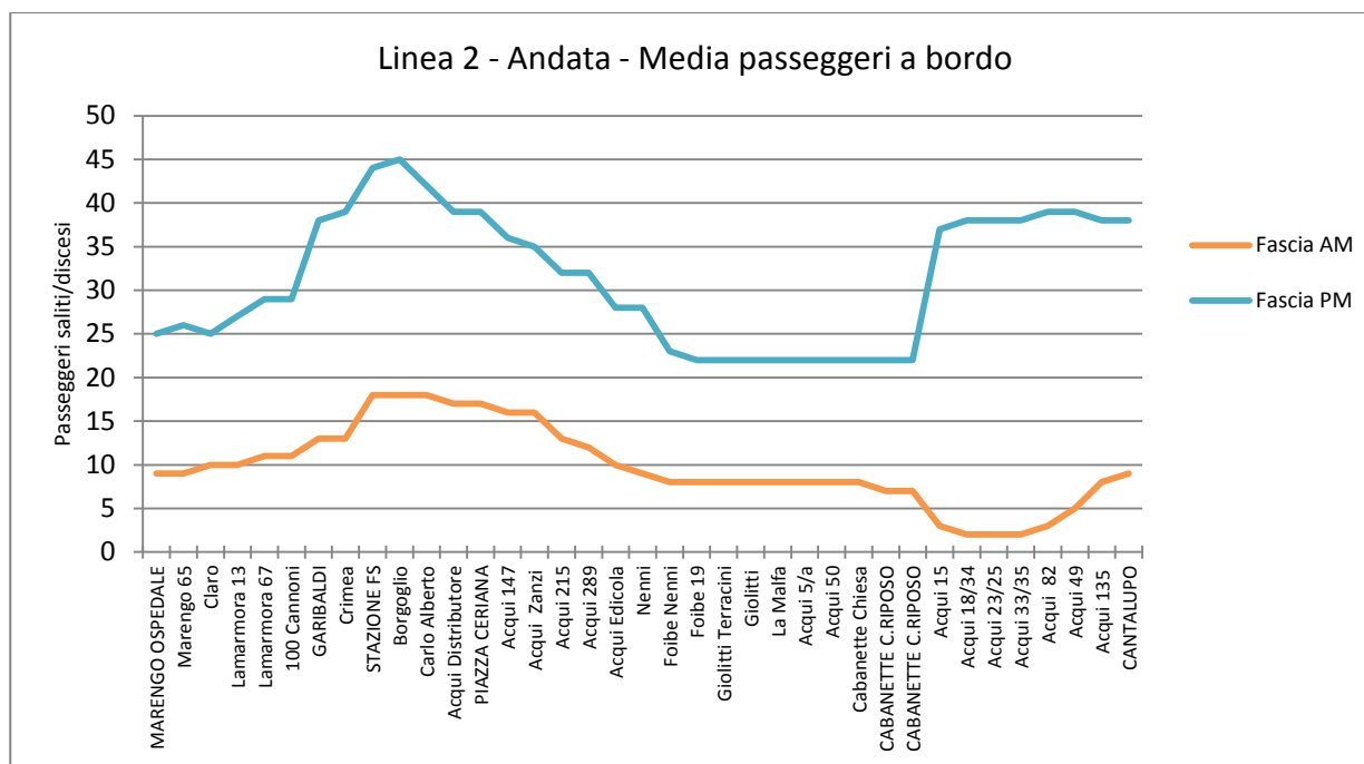
Figura 4-20: Utilizzo fermate. Totale passeggeri corse di andata per fascia oraria. Linea 2
