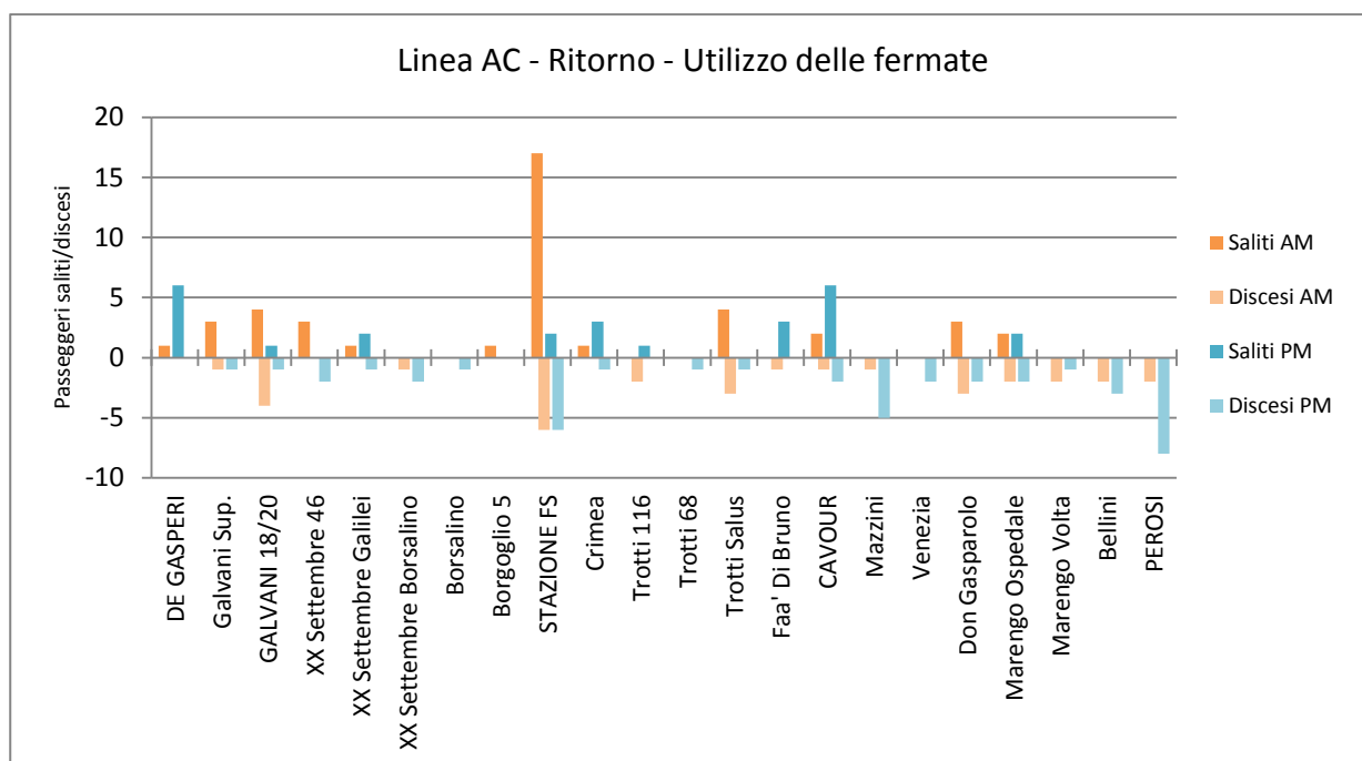
Figura 4-15: Utilizzo fermate. Totale passeggeri corse di ritorno per fascia oraria. Linea A/C
