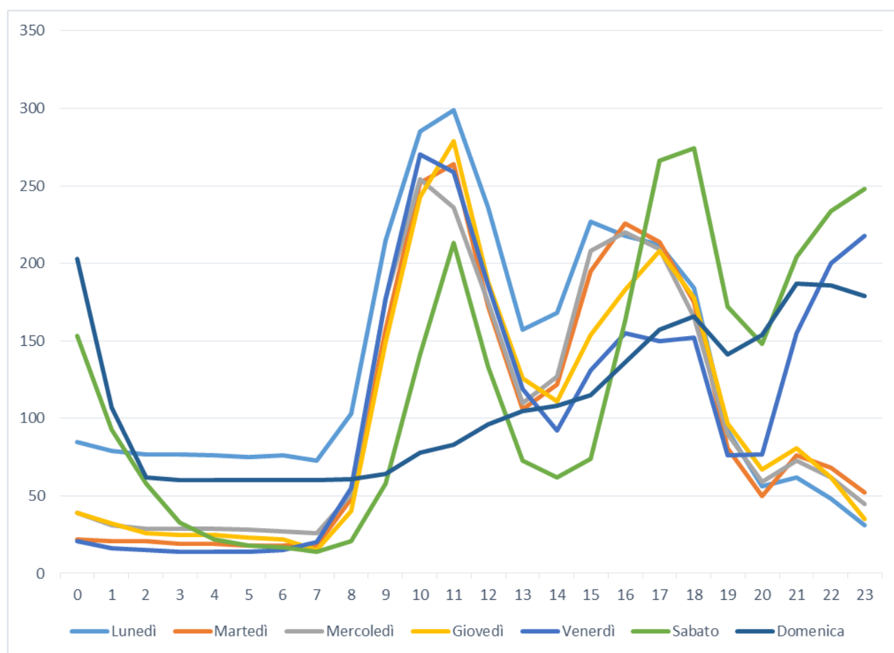
Figura 5-7: Parcheggio Piazza Libertà: numero medio di auto in sosta per ora e per giorno della settimana (aprile 2016)
