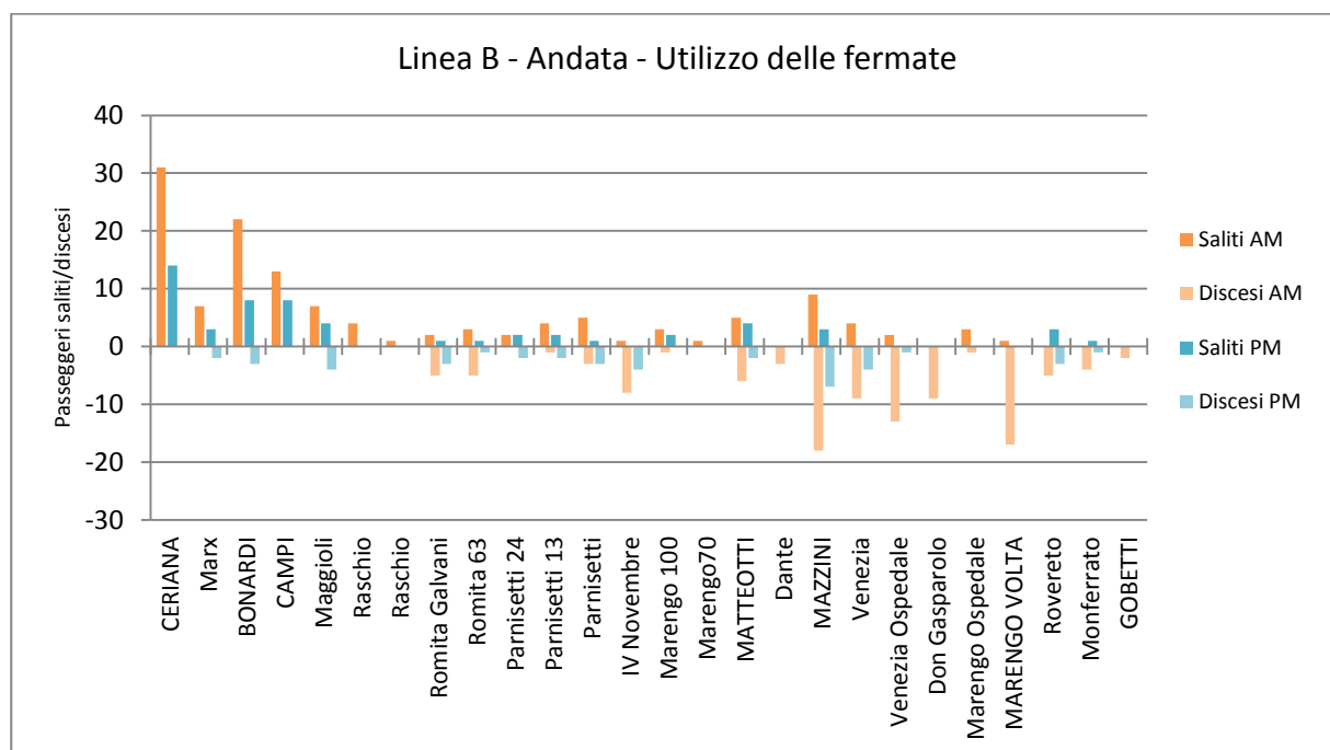
Figura 4-17: Utilizzo fermate. Totale passeggeri corse di andata per fascia oraria. Linea B
